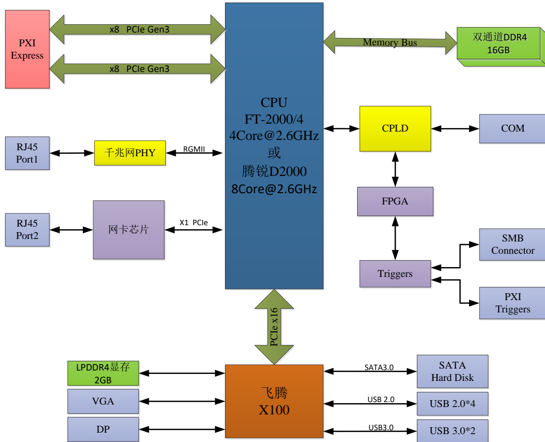
图 1-1 系统功能框图
