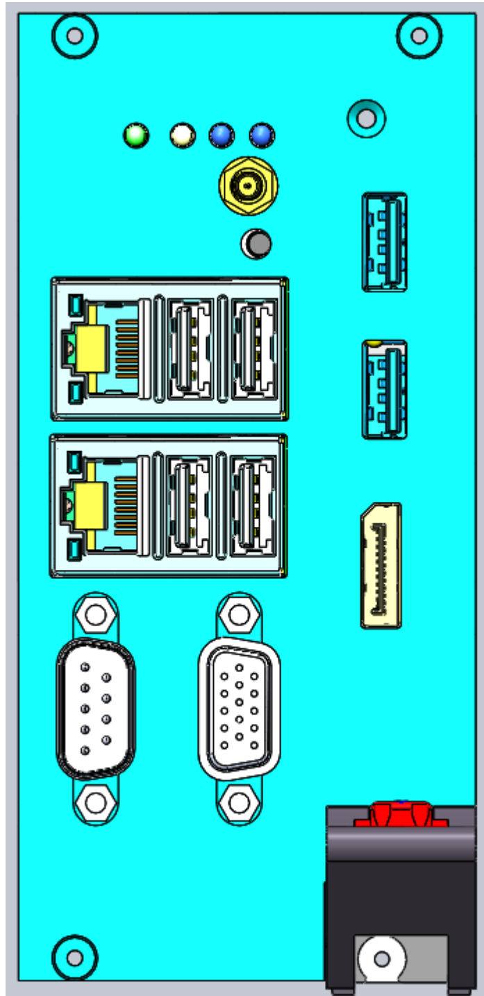
图 2-1 PXIe-63860 产品面板布局图
