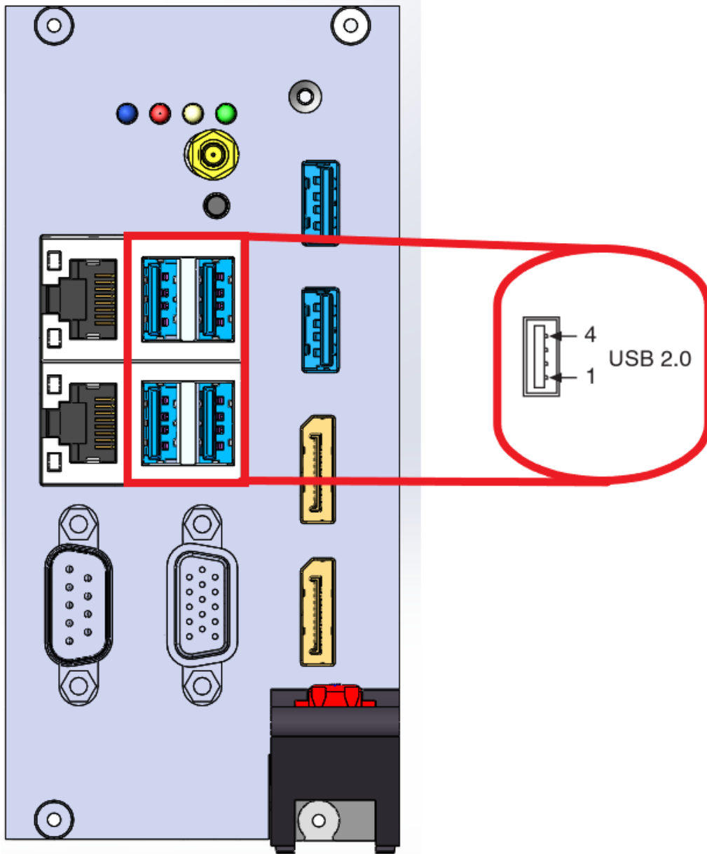
图 3-7 USB2.0 接口示意图
