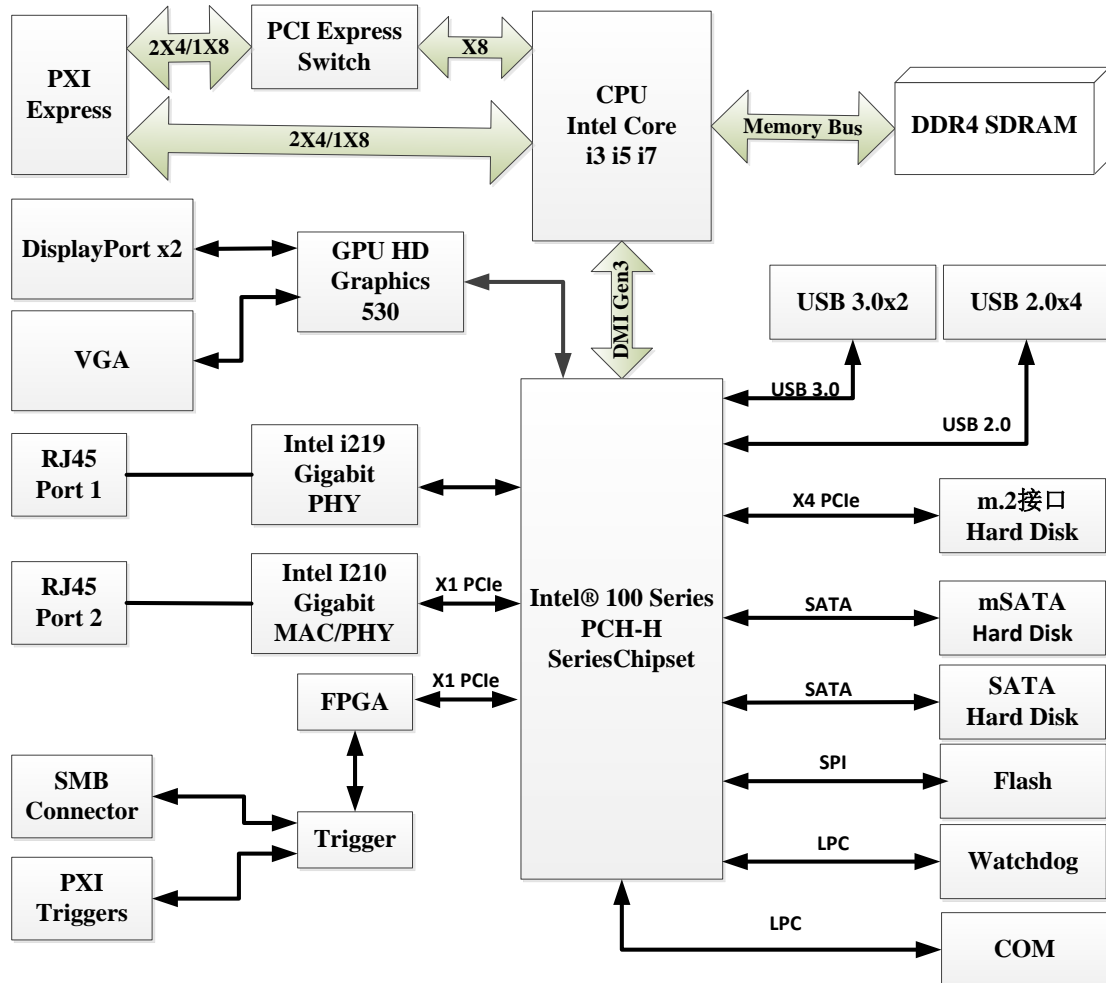
图 1-2 搭载 i7-6820EQ/6822EQ、i5-6440EQ、i3-6100E CPU 系统功能框图
