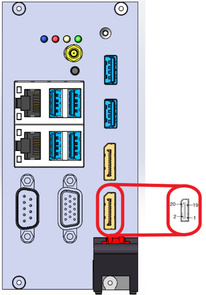
图 3-2 DP 接口 2 示意图
