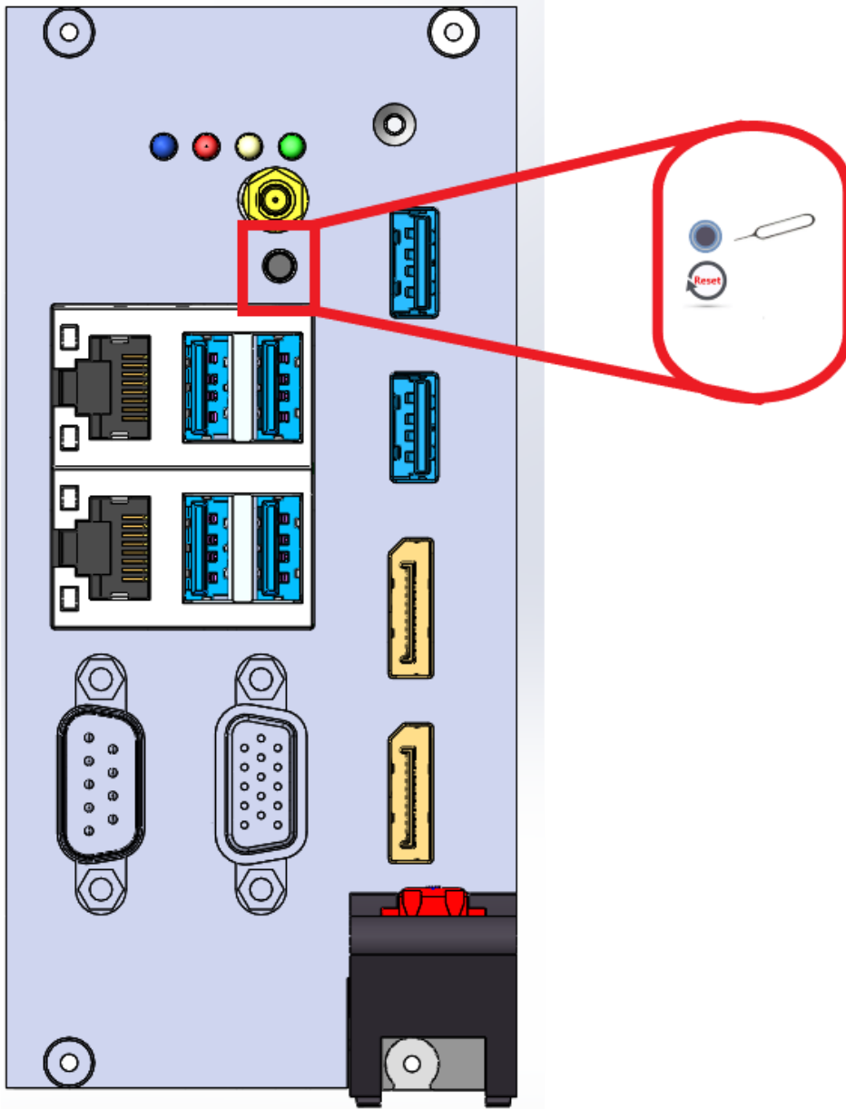
图 3-9 复位接口示意图
