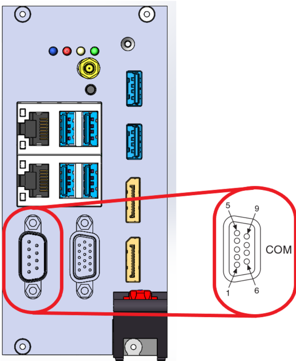
图 3-4 COM 接口示意图
