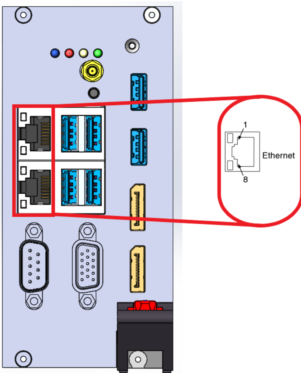
图 3-5 以太网接口示意图
