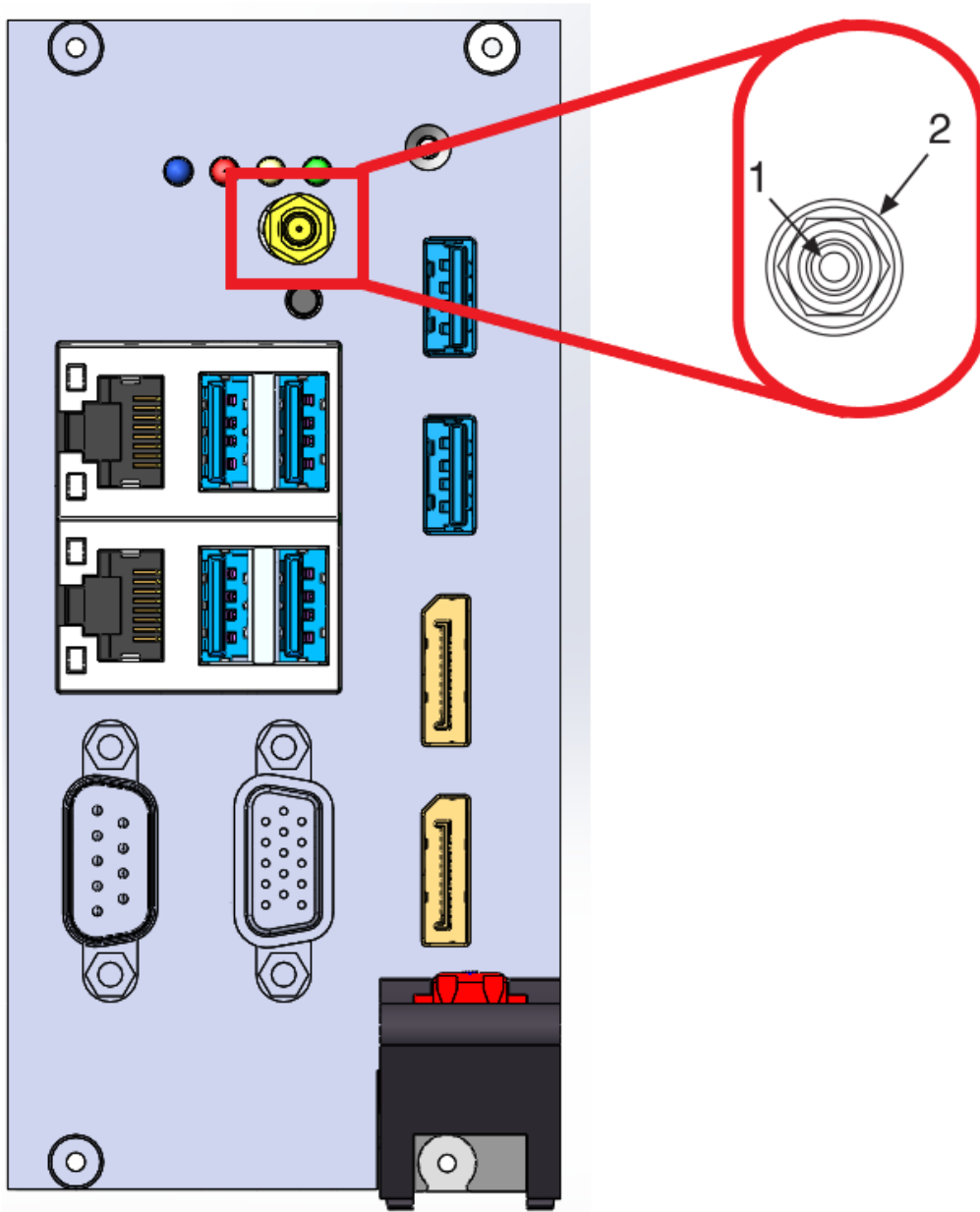
图 3-8 触发接口示意图
