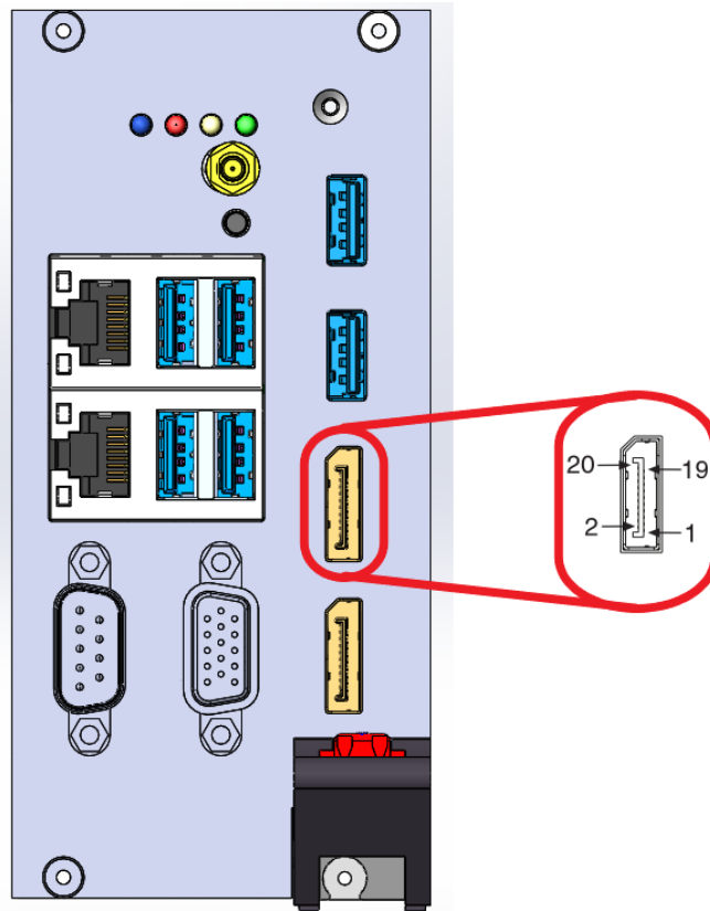
图 3-1 DP 接口 1 示意图
