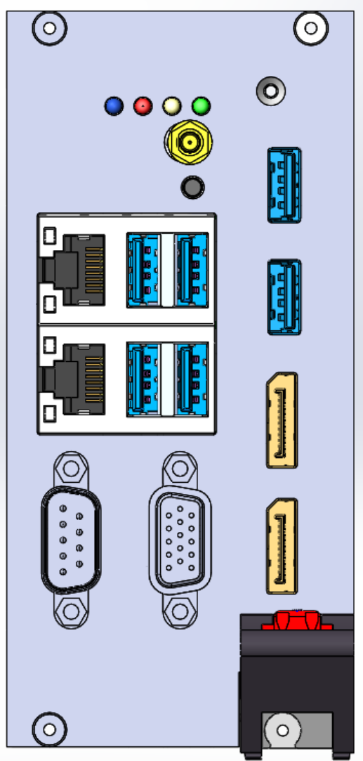
图 2-2 PXIe-3876 产品面板布局图
