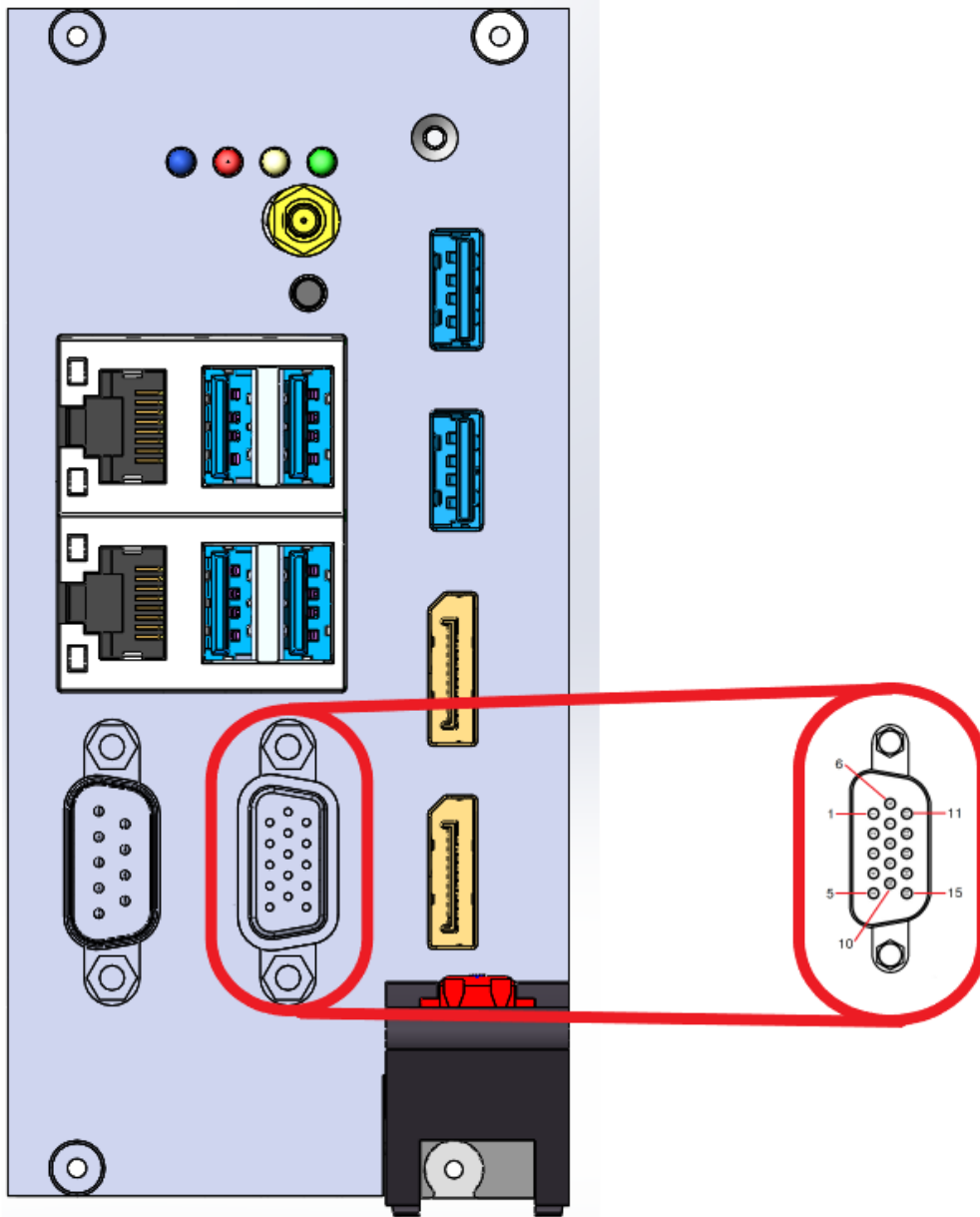
图 3-3 VGA 接口示意图
