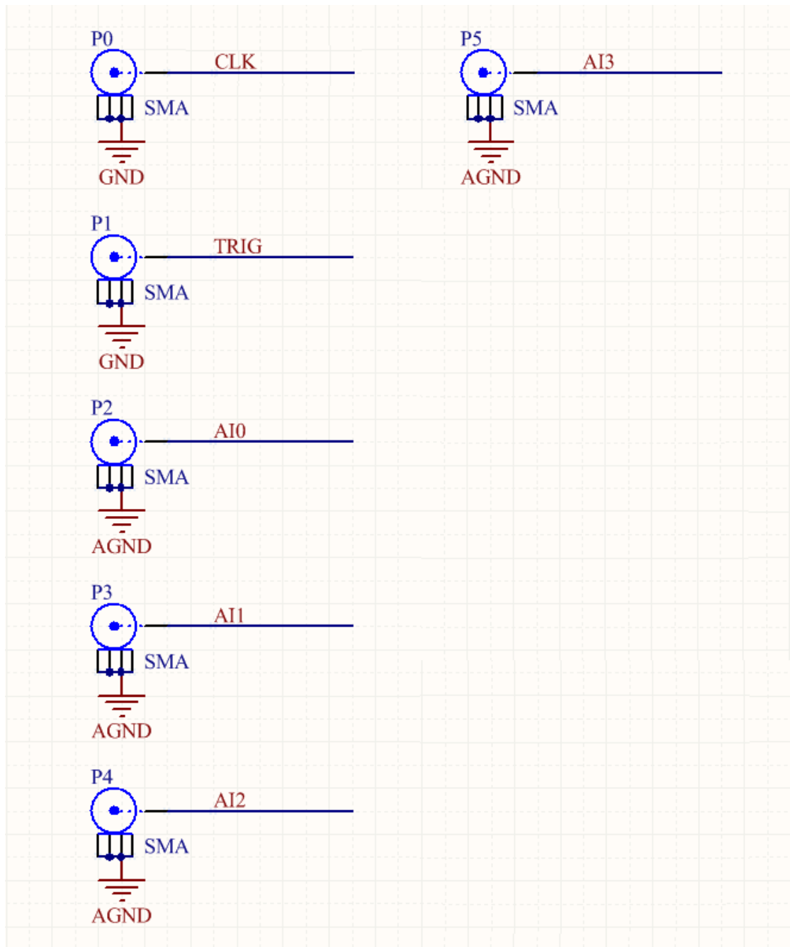
图 3-2 SMB 接口定义
