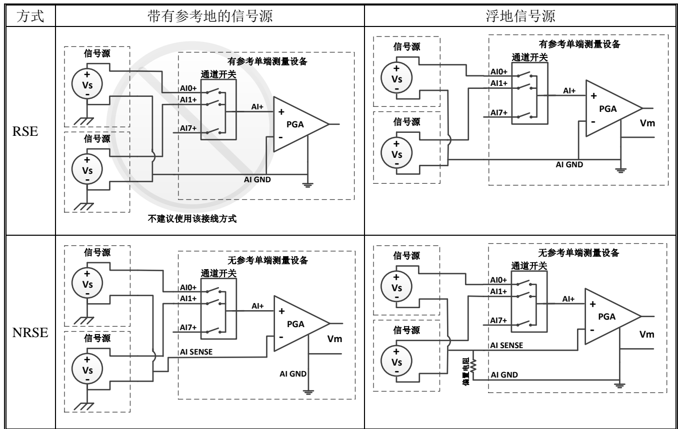
图 3-5 单端连接方式
