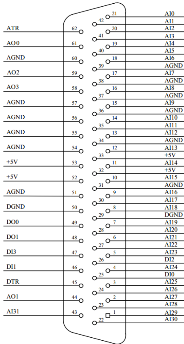
图 3-2 62 芯 D 型连接器示意图
