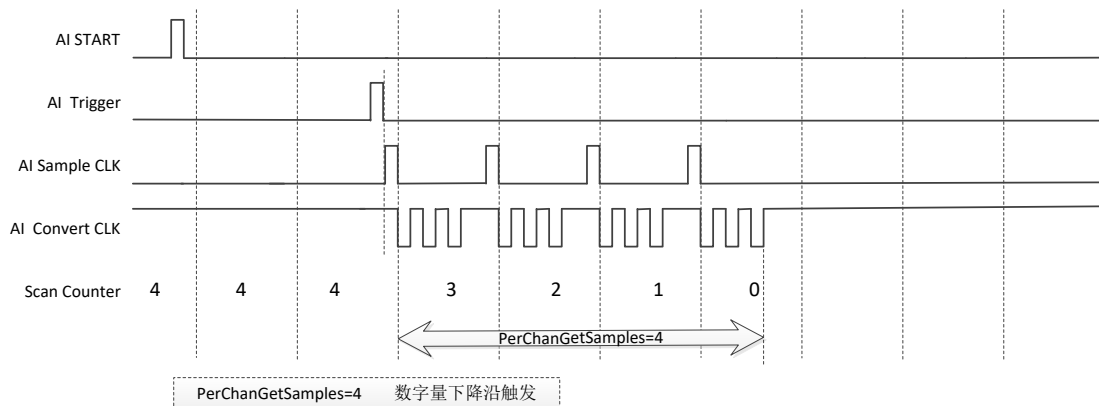
图 4-1 后触发模式
