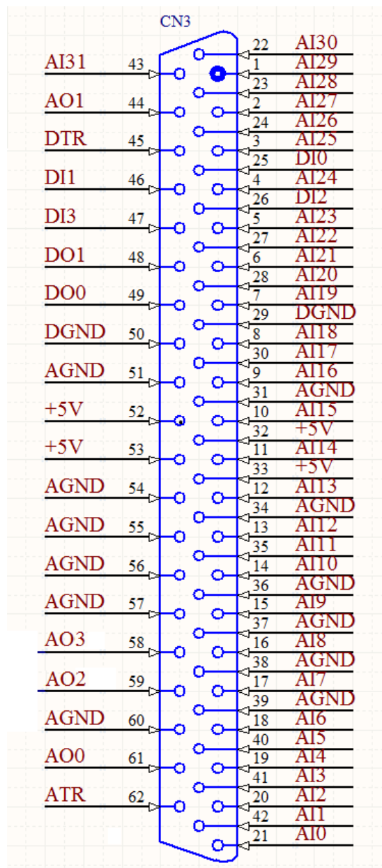
图 3-1 板卡左侧 62 芯 D 型连接器原理图
