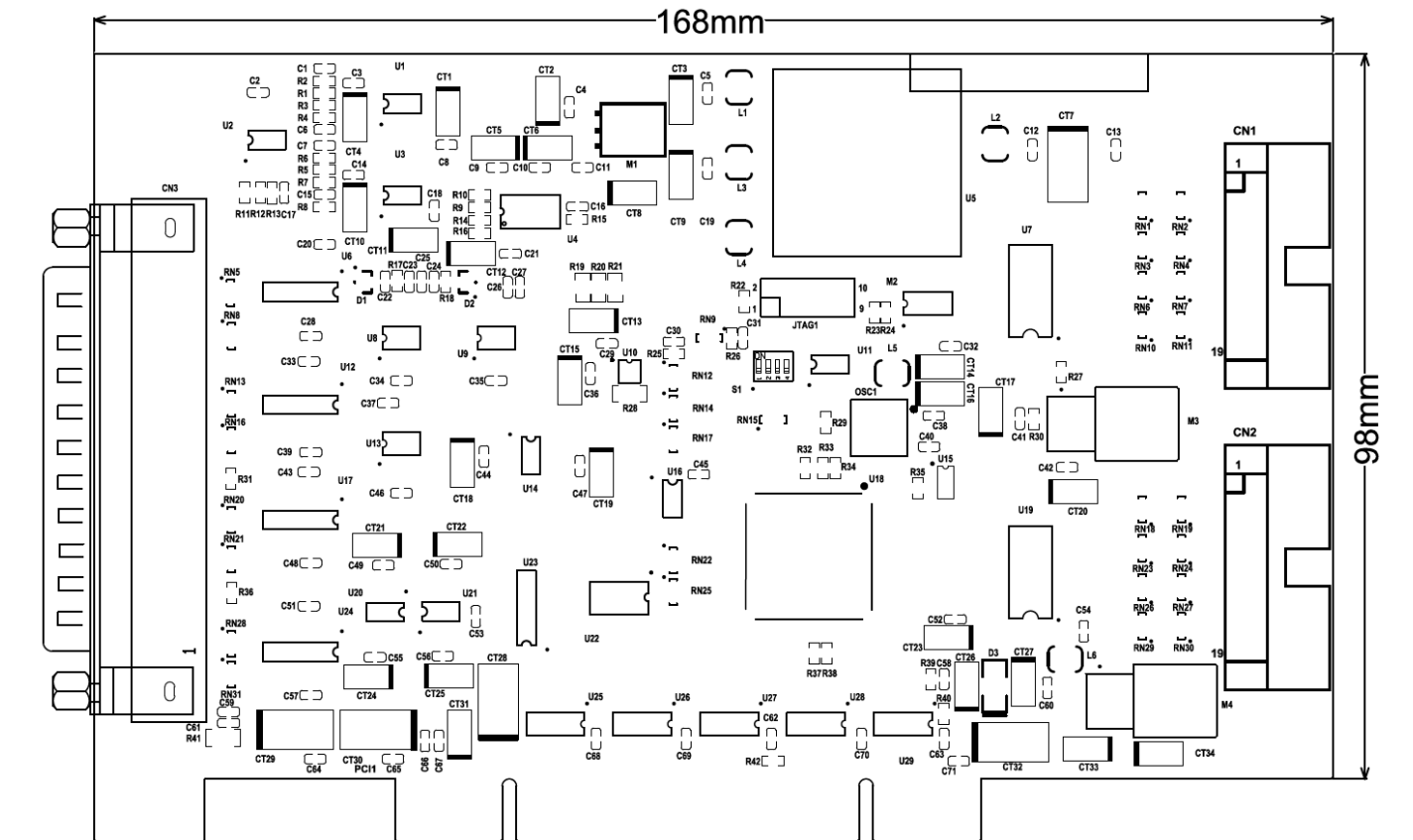
图 2-1 产品布局图
