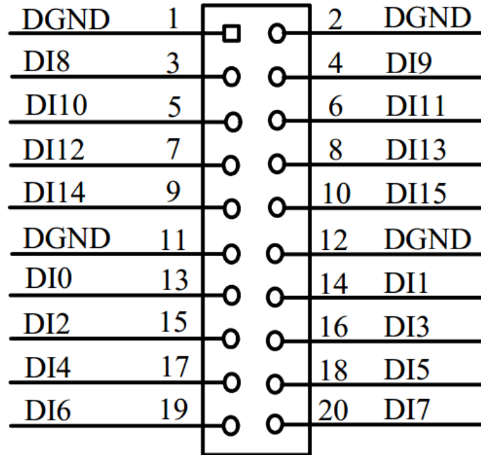
图 3-3 20P 连接器(CN1)端子示意
