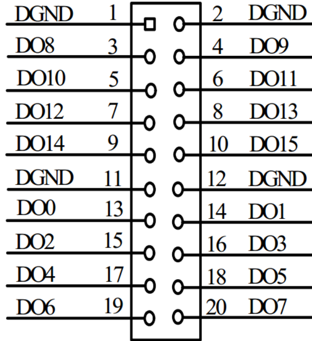
图 3-4 20P 连接器(CN2)端子示意
