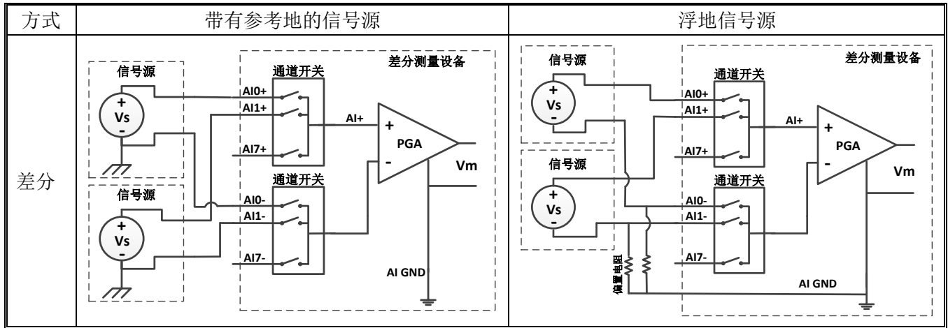
图 3-6 差分连接方式
