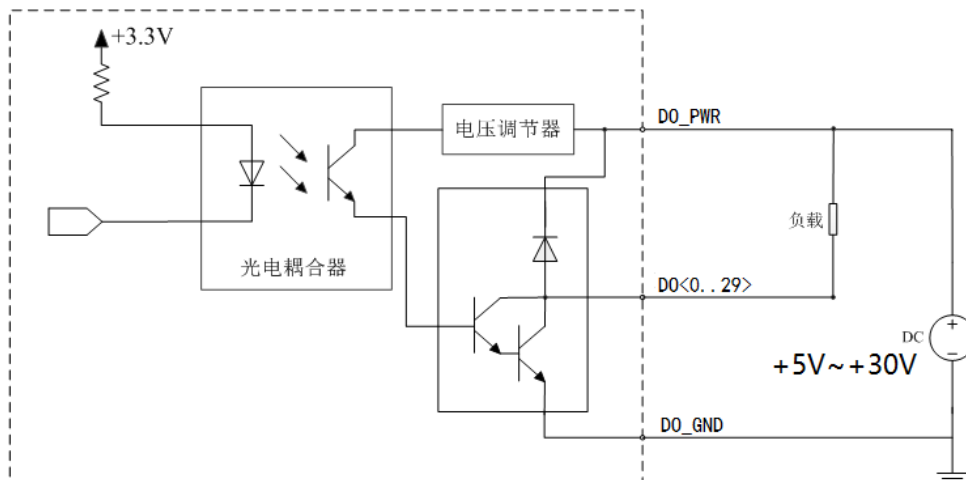
图 3-5 数字量输出接线示意
