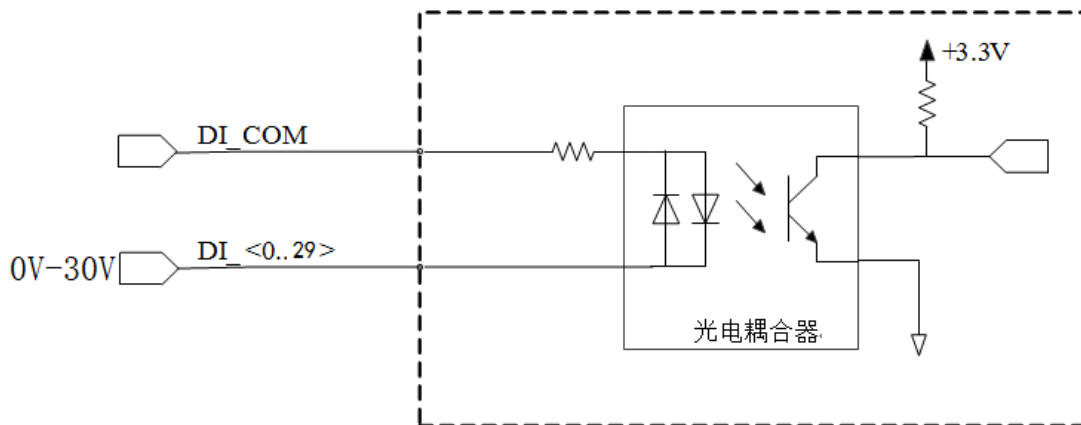
图 3-3 数字量输入接线示意
