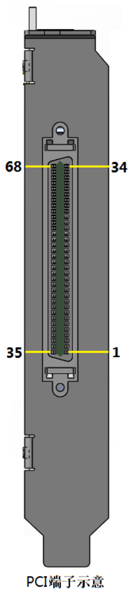
图 3-1 板卡接线端子示意图
