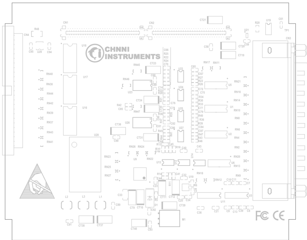
图 2-1 NET6268 产品布局图
