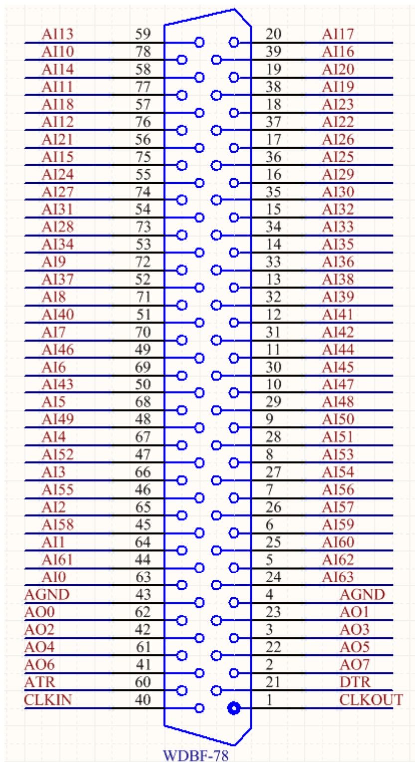
图 3-1 78 芯 D 型头端子示意图
