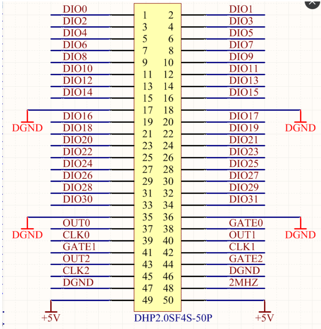
图 3-2 线缆焊接头标注
